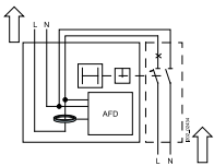
5SM6011-1
