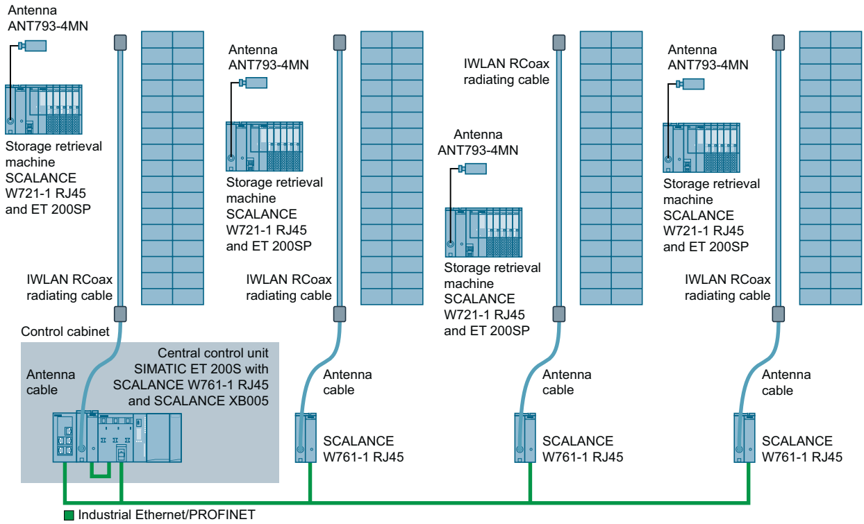
Rcoax kablosuz haberleşme sistemi örneği
